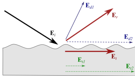
Рис. 2. Полный набор электромагнитных волн в задаче о возбуждении поверхностного плазмона падающим оптическим излучением. Жирными векторами показаны волновые вектора полей нулевого порядка малости, тонкими – первого
