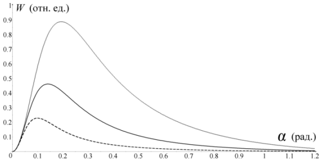
Рис. 1. Теоретическая зависимость энергии ТГц излучения от угла падения оптического импульса для металлов с разной концентрацией свободных электронов. Сдвиг максимума вправо соответствует уменьшению плазменной частоты, графики соответствуют плазменной частоте, в 5, 7 и 10 раз большей частоты лазерного излучения
