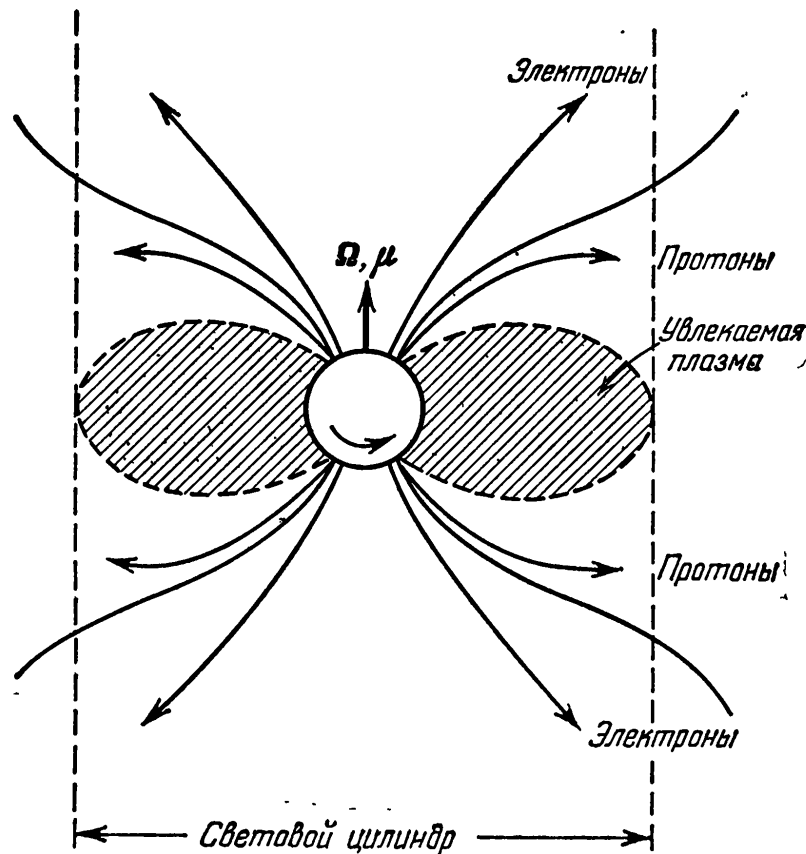
Рис. 5. Модель магнитосферы нейтронной звезды [8].
