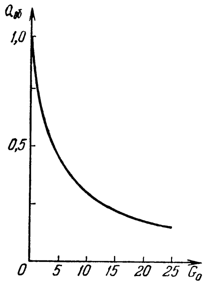
Рис. 27. Коэффициент трансформации Q_{об} при прохождении волн через область с нулевым магнитным полем (зависимость от параметра взаимодействия G_0 )
