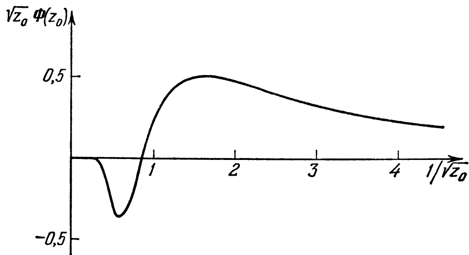
Рис 58. График зависимости V z_0 \Phi(z_0) от 1/V z_0 .
