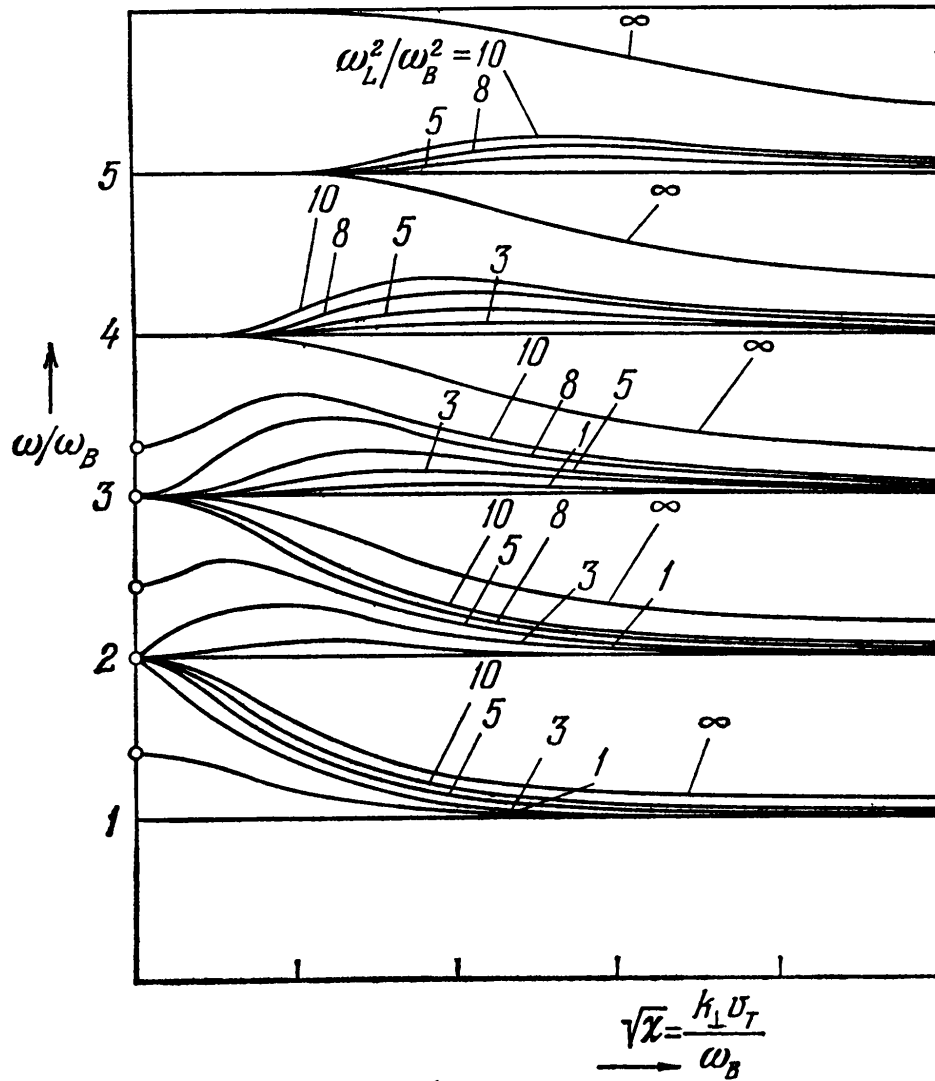
Рис. 15. Дисперсионные кривые для мод Бернштейна в нерелятивистской равновесной плазме. Светлыми точками на оси \omega/\omega_B отмечены значения, где \omega = \omega_r .
