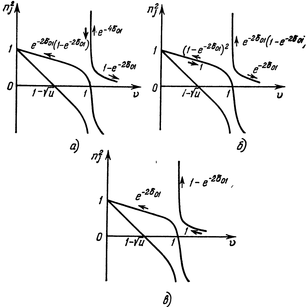
Рис. 33. Различные варианты (а, б и в) линейного взаимодействия волн при u = \omega_B^2 / \omega^2 < 1 . Указаны квадраты модулей амплитуд волн, выходящих из области взаимодействия, при падении на нее волны с единичной амплитудой. Жирной стрелкой отмечена падающая волна, тонкими стрелками — волны, возникающие в результате взаимодействия.
