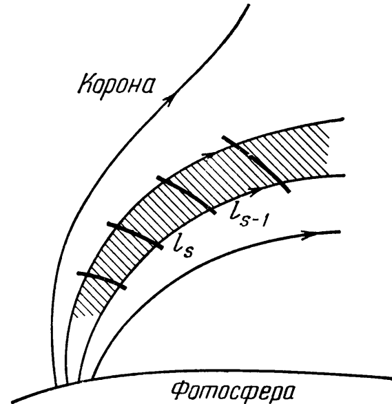
Рис. 54. Модель распределенного источника для солнечного радиоизлучения, обладающего «зеебра»-структурой. Область, занимаемая энергичными электронами, заштрихована ( l — координата вдоль силовой трубки).
