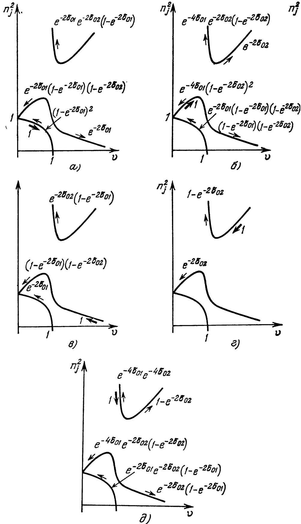
Рис. 34. Различные варианты линейного взаимодействия при u \cos^2 \alpha > 1 . Обозначения те же, что на рис. 33.
