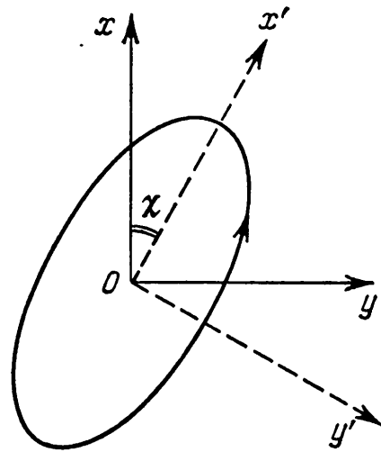
Рис 6. Эллипс поляризации для излучения с волновым вектором k , направленным за чертеж
