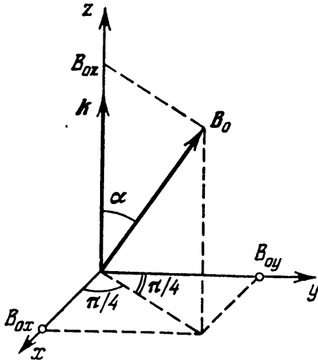
Рис. 28. Координатная система III .
