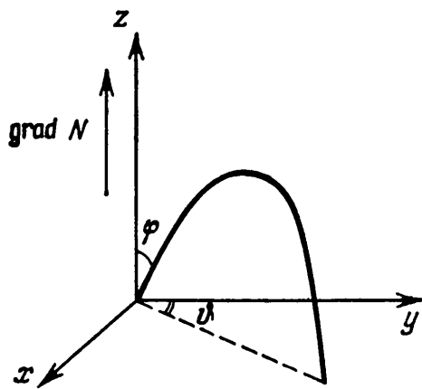
Рис. 35. К учету рефракции в уравнении переноса излучения в плоскослоистой среде.
