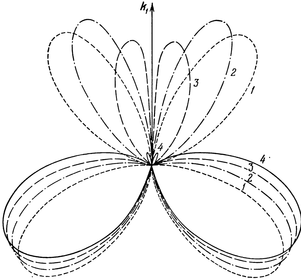
Рис. 62. Диаграмма направленности радиоизлучения \Psi(\theta_0) на второй гармонике плазменной частоты в однородной плазме: 1 — v_\phi/c = 0,2 ; 2 — v_\phi/c = 0,4 ; 3 — v_\phi/c = 0,6 ; 4 — v_\phi/c = 0,8 .
