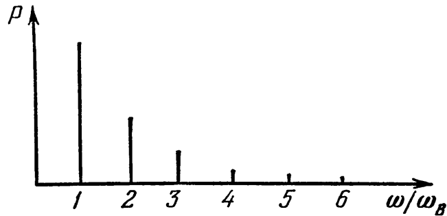
Рис. 39. Частотный спектр циклотронного излучения электрона в вакууме.
