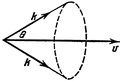
Рис. 37. Конус волновых векторов при эффекте Вавилова — Черенкова.
