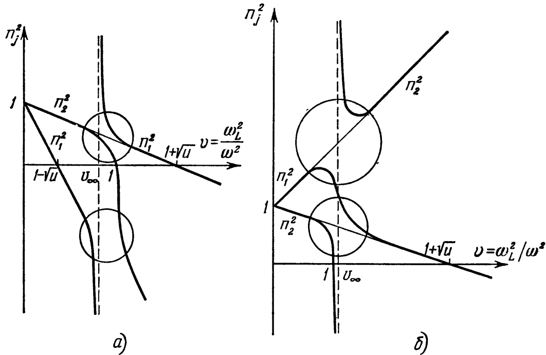
Рис. 11. Зависимость n_j^2(v) при \alpha \ll 1 : а) u < 1 ; б) u \cos^2 \alpha > 1 . Крестками отмечены области линейного взаимодействия волн (см. § 7).
