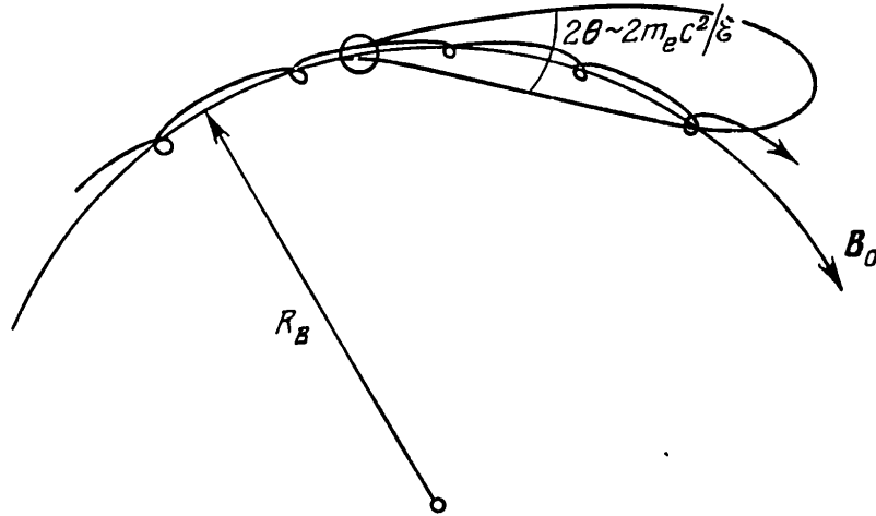
Рис 42 Мгновенная диаграмма направленности излучения из-за кривизны силовых линий ( R_B — радиус кривизны).
