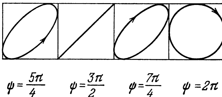
Рис. 36. Изменение характера поляризации излучения с ростом разности фаз \psi : а) эффект Фарадея ( a=b , \rho=1 ); б) эффект Коттона — Мутона ( a=b , \rho=0 ).
