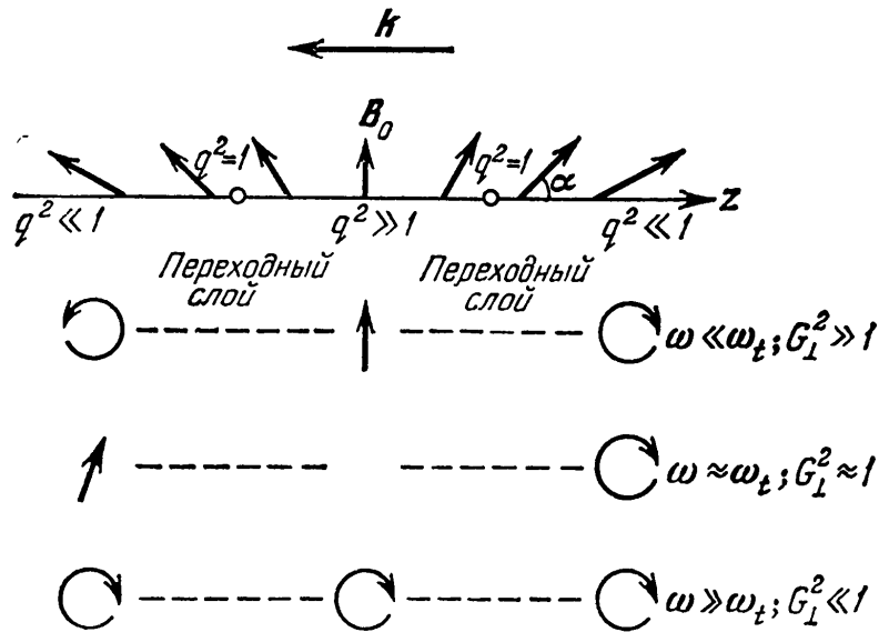
Рис. 24 Распространение волн через область квазипоперечного магнитного поля и изменение их поляризации.
