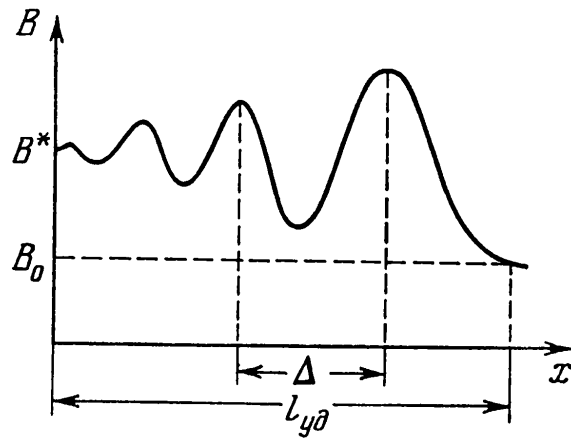
Рис. 48 Профиль ударной волны в плазме.
