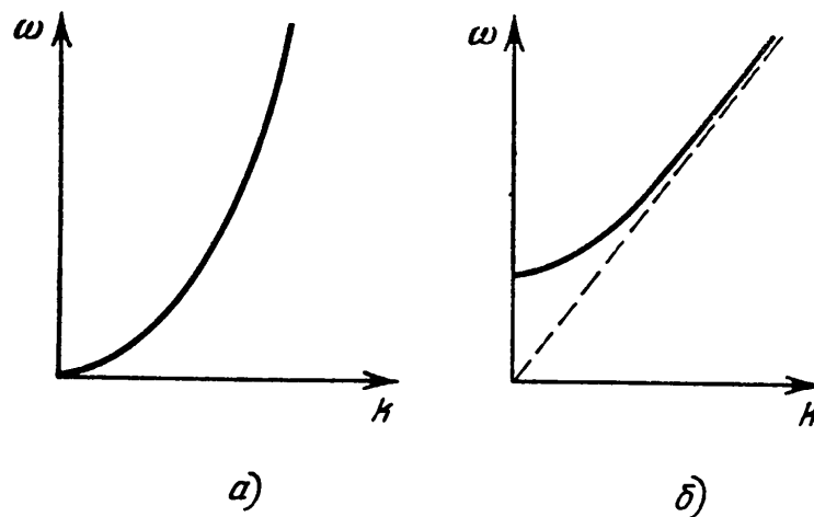
Рис 59. Примеры распадного (а) и нераспадного (б) спектров
