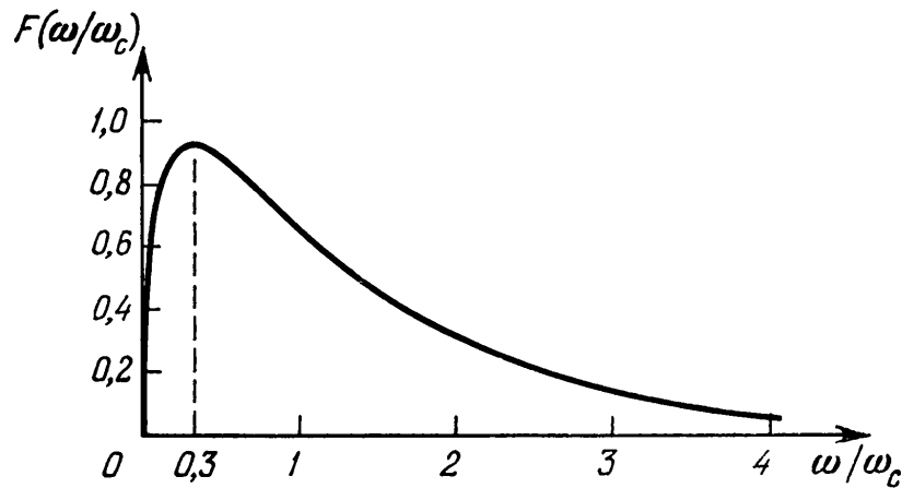
Рис. 40. Частотный спектр синхротронного излучения электрона в вакууме.
