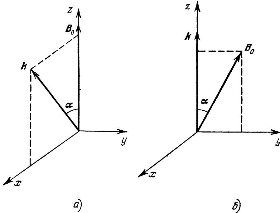
Рис. 7. Ориентация векторов B_0 и k относительно координатных осей: а) система координат I; б) система координат II
