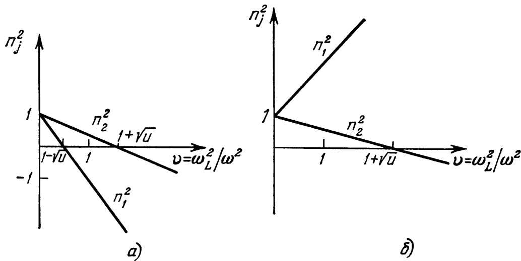
Рис. 9. Зависимость n_j^2(v) при продольном распространении в магнитном поле: а) u < 1 ; б) u > 1
