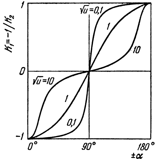
Рис. 13. Коэффициент поляризации K_{1,2} в функции угла \alpha .
