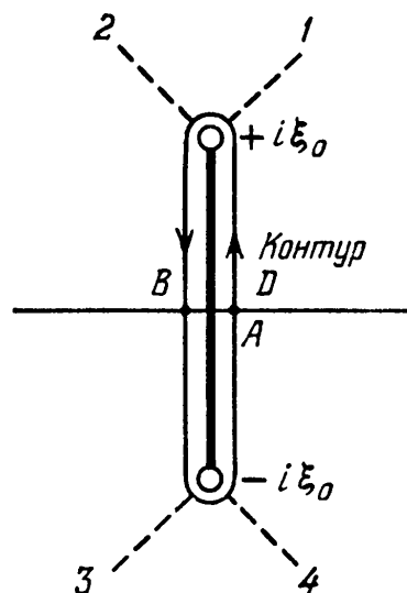
Рис. 30. Расположение линий Стокса на комплексной плоскости \xi для n_2 - n_1 = \sqrt{\xi^2 + \xi_0^2} (пунктирные линии 1—4).
