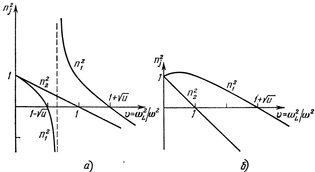
Рис 10 Зависимость n_j^2(\nu) при поперечном распространении волн в магнитном поле: а) u < 1 ; б) u > 1
