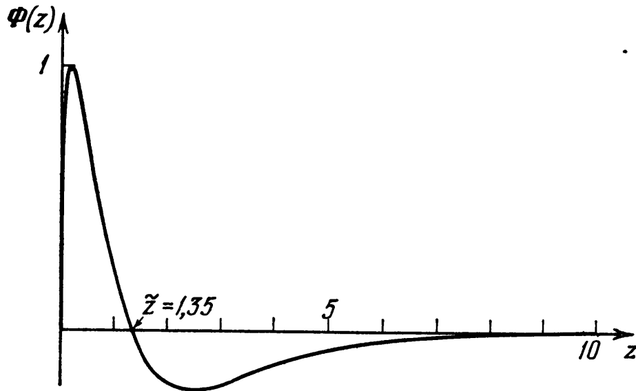
Рис. 57. График функции \Phi(z) .
