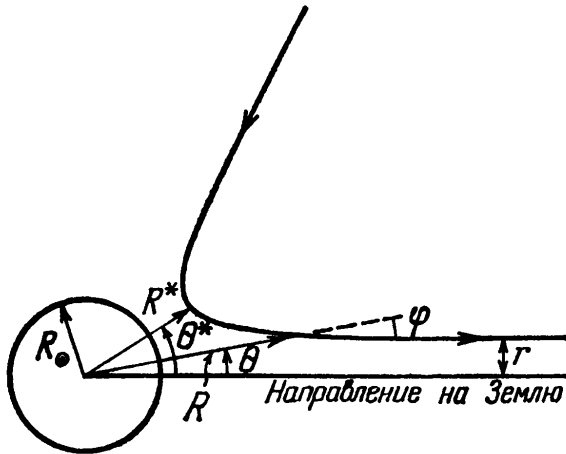
Рис. 21. К расчету формулы луча в сферически-симметричной солнечной короне.
