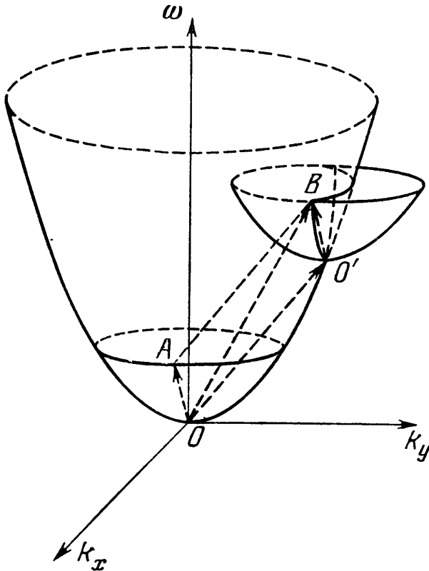
Рис. 60. Критерий распадного спектра
