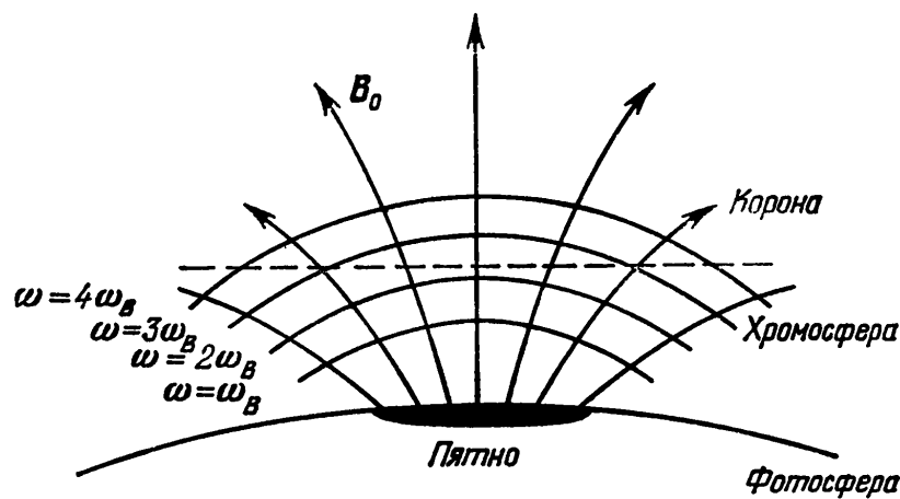
Рис 45. Расположение гирорезонансных уровней в униполярном магнитном поле.
